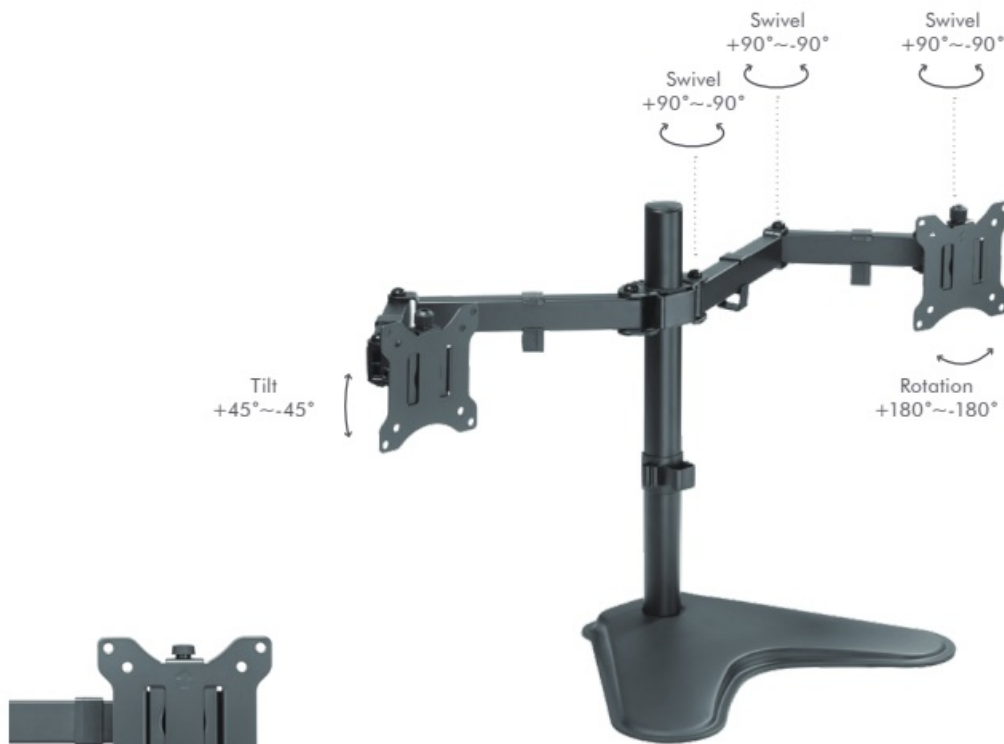
Detachable VESA Plate
