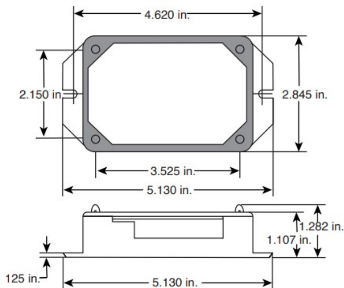
Mini Meter Case and Cover Dimensions
