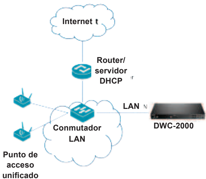
Figura 10. Topología de la red
