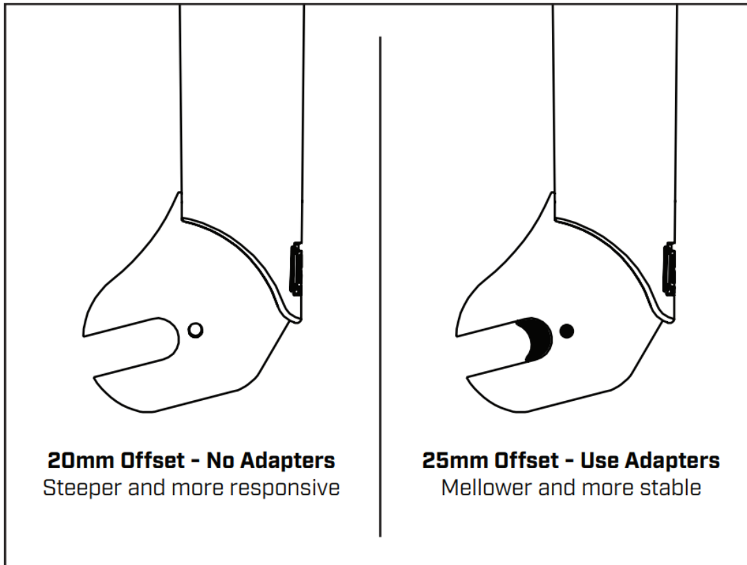
FIG. 1 - OFFSET OPTIONS
