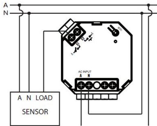
FUNCTION 1 - TOGGLE INPUT
