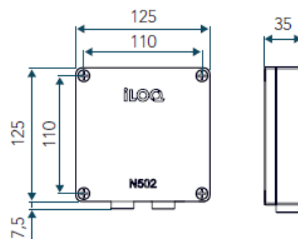
iLOQ N501 4G Standalone Door Module & iLOQ N502 Online Door Module
