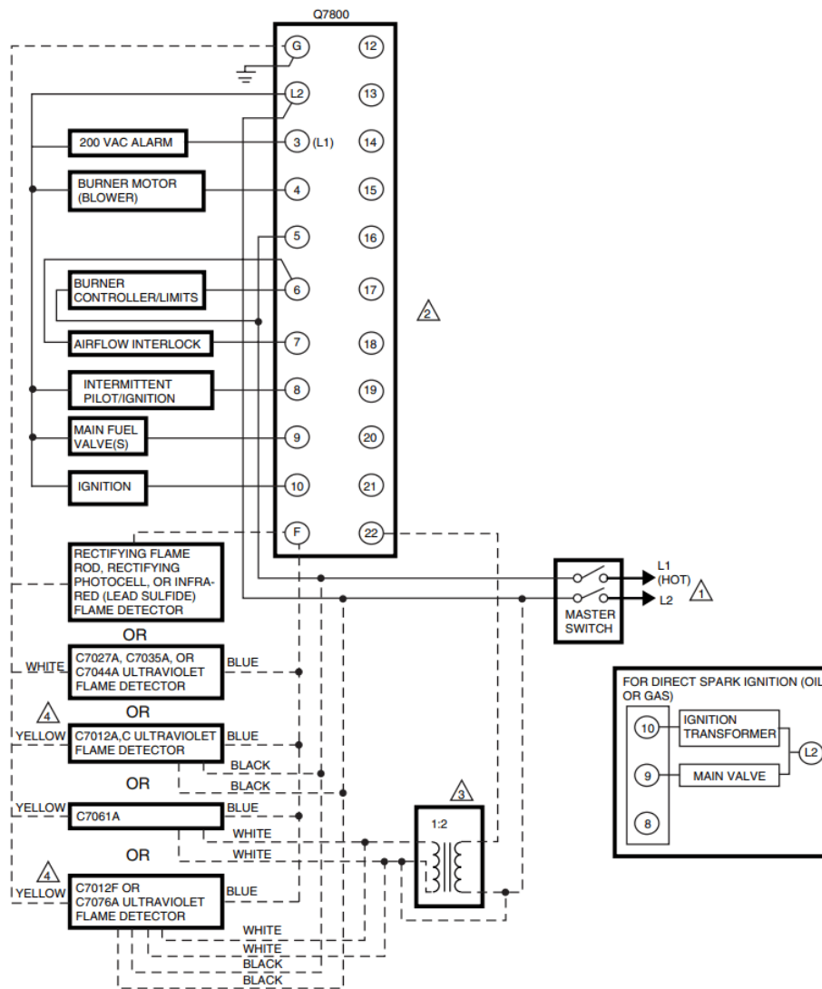
Fig. 8. Wiring the EC7895.
