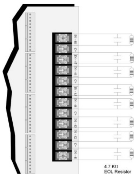
Input Wiring
