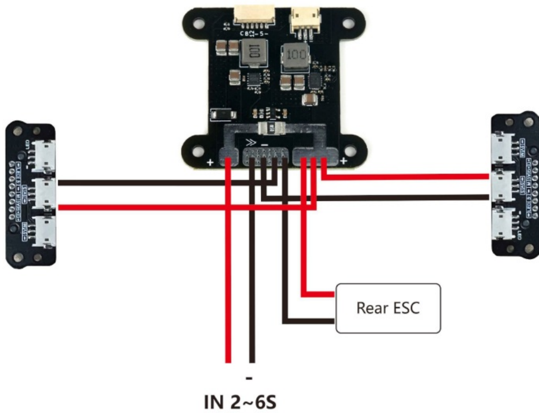
Master Wiring
