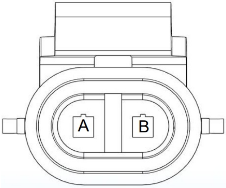
Solenoid 2 Plug on Baler Harness 006-765B2 (Deutsch Plug Number: APTIV 12052641)
