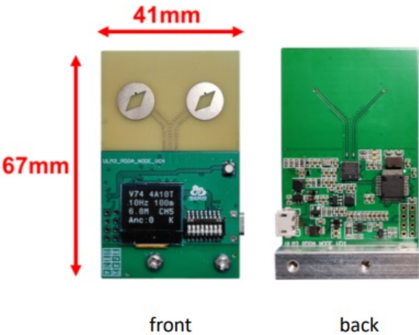
Pic 5-1 ULM3-PDOA Module
