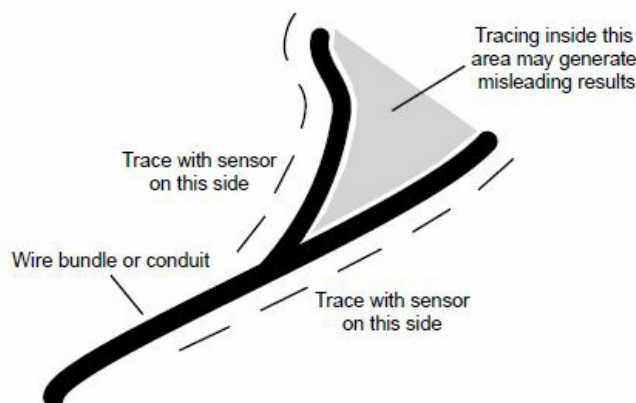
Fig. 8 - Tracing Wires inside bundles and conduits
