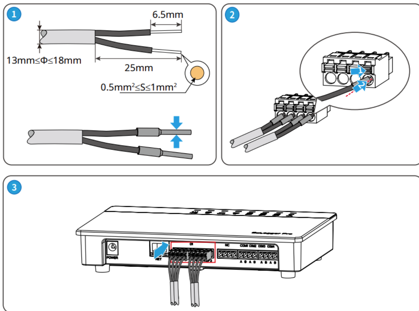
Figure 4.4-3 Wiring of EzLogger Pro DI port
