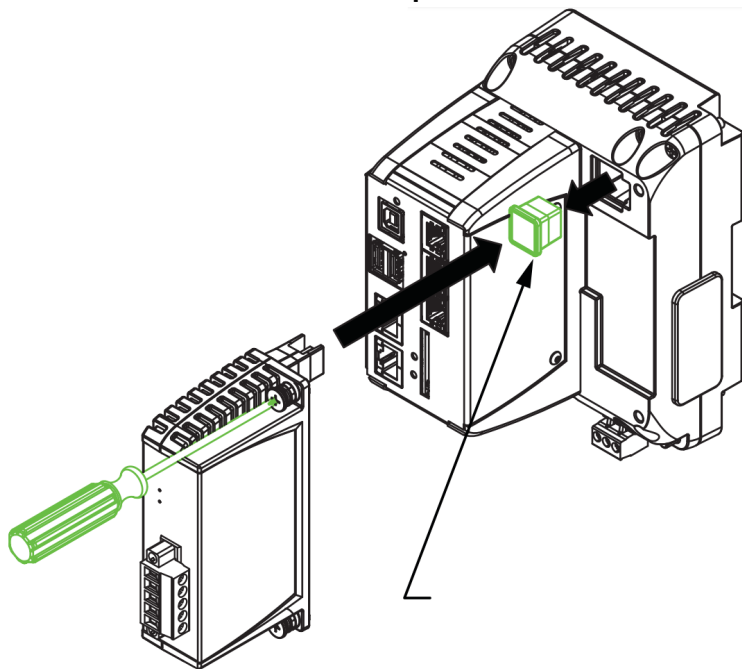
REMOVE RUBBER MODULE PLUG
