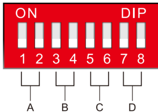
EQ DIP-SWITCHES
