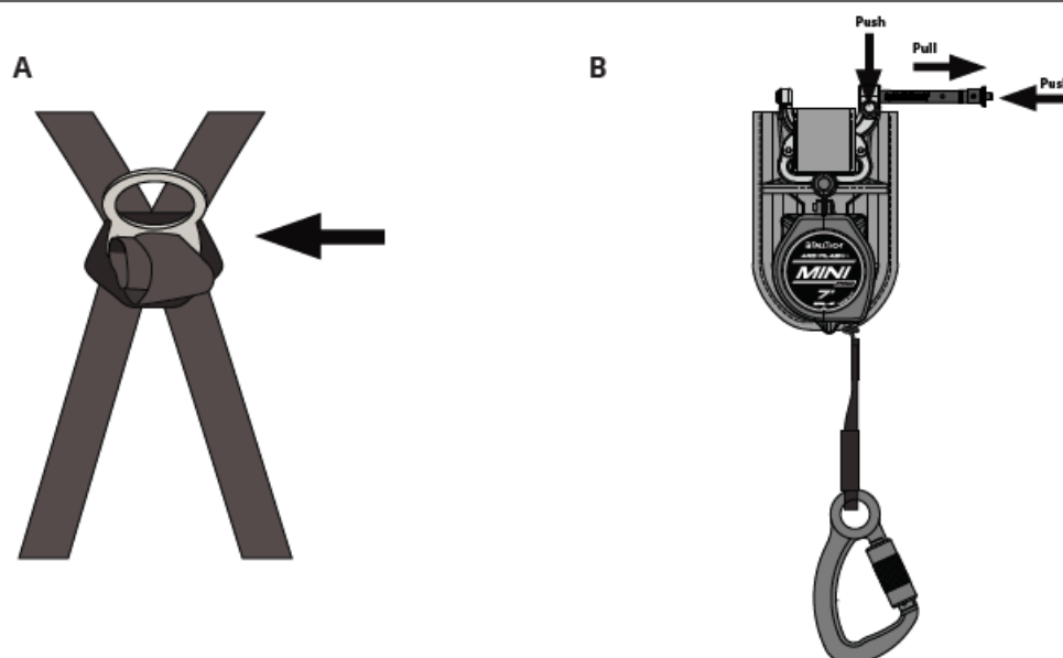
Figure 3 - Arc Flash Mini Pro SRL-P Installation
