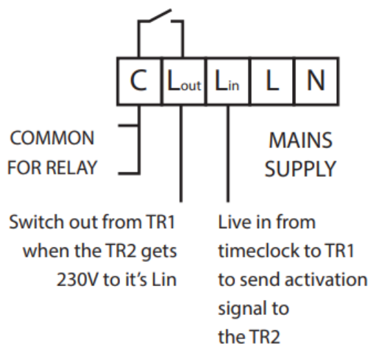
Internal wiring diagram TR1
