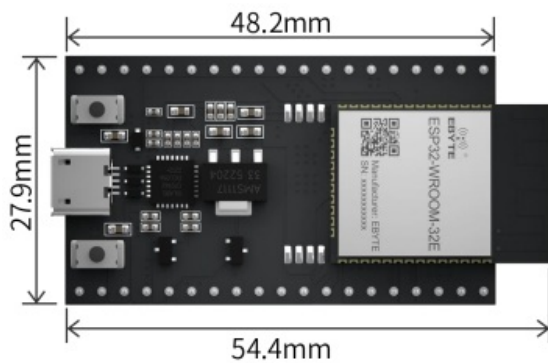
ESP32-WROOM-32E
