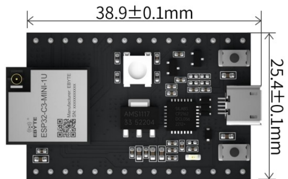
ESP32-C3-MINI-1U-TB
