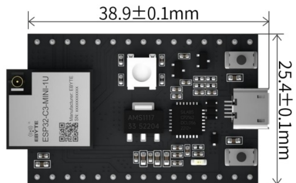
ESP32-C3-MINI-1U-TB
