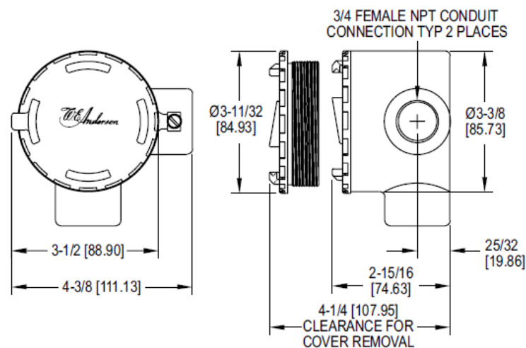
CSA, IECEx, ATEX conduit enclosure
