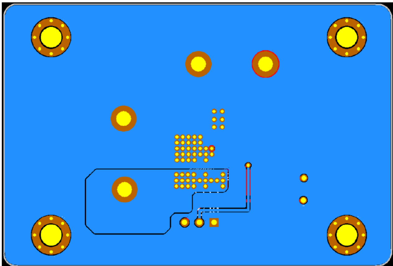
Figure 4. AP61302QZ6 - EVM - Bottom Layer
