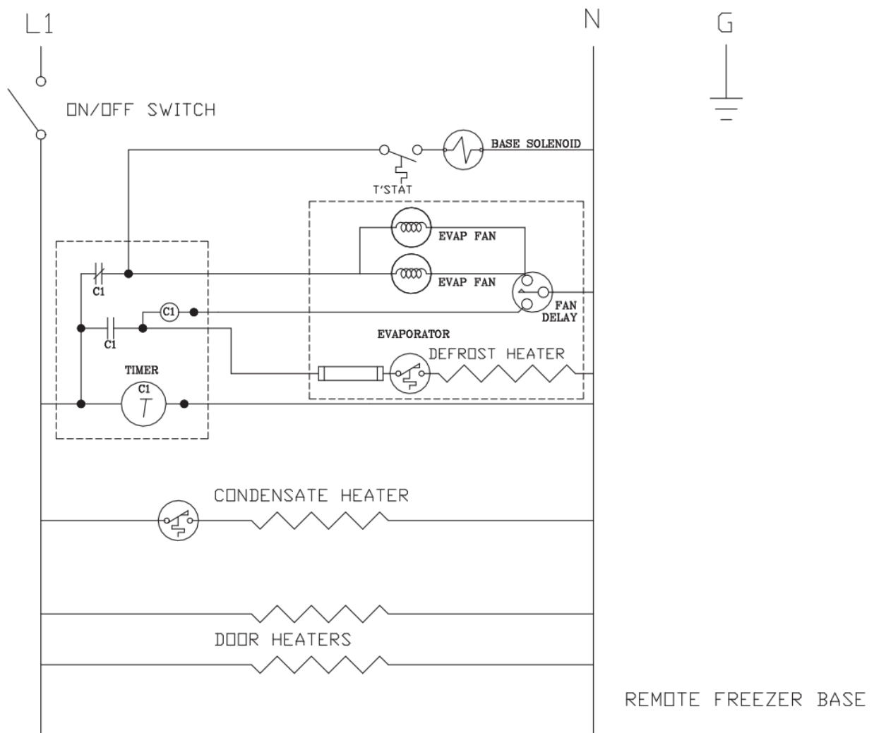
Wiring Diagram, F18FR
