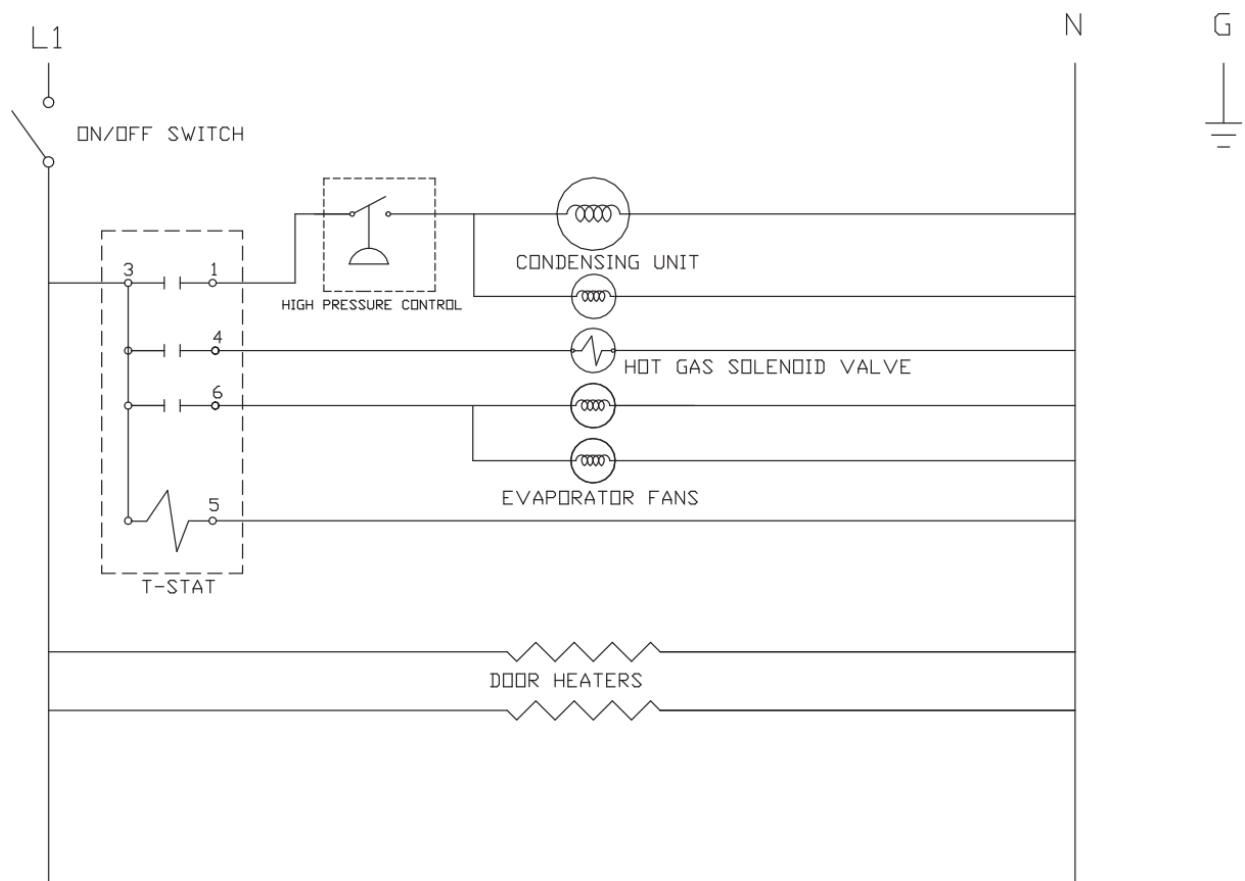
Wiring Diagram, F18FR
