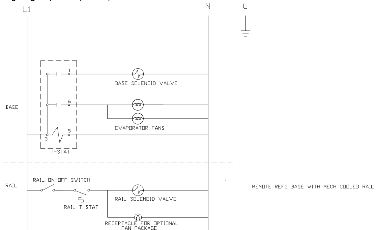
Wiring Diagram, F18MR, F18SR, F18DR & F18RR
