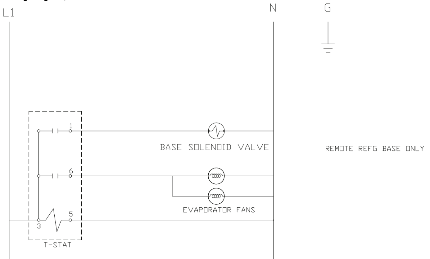
Wiring Diagram, F18WR
