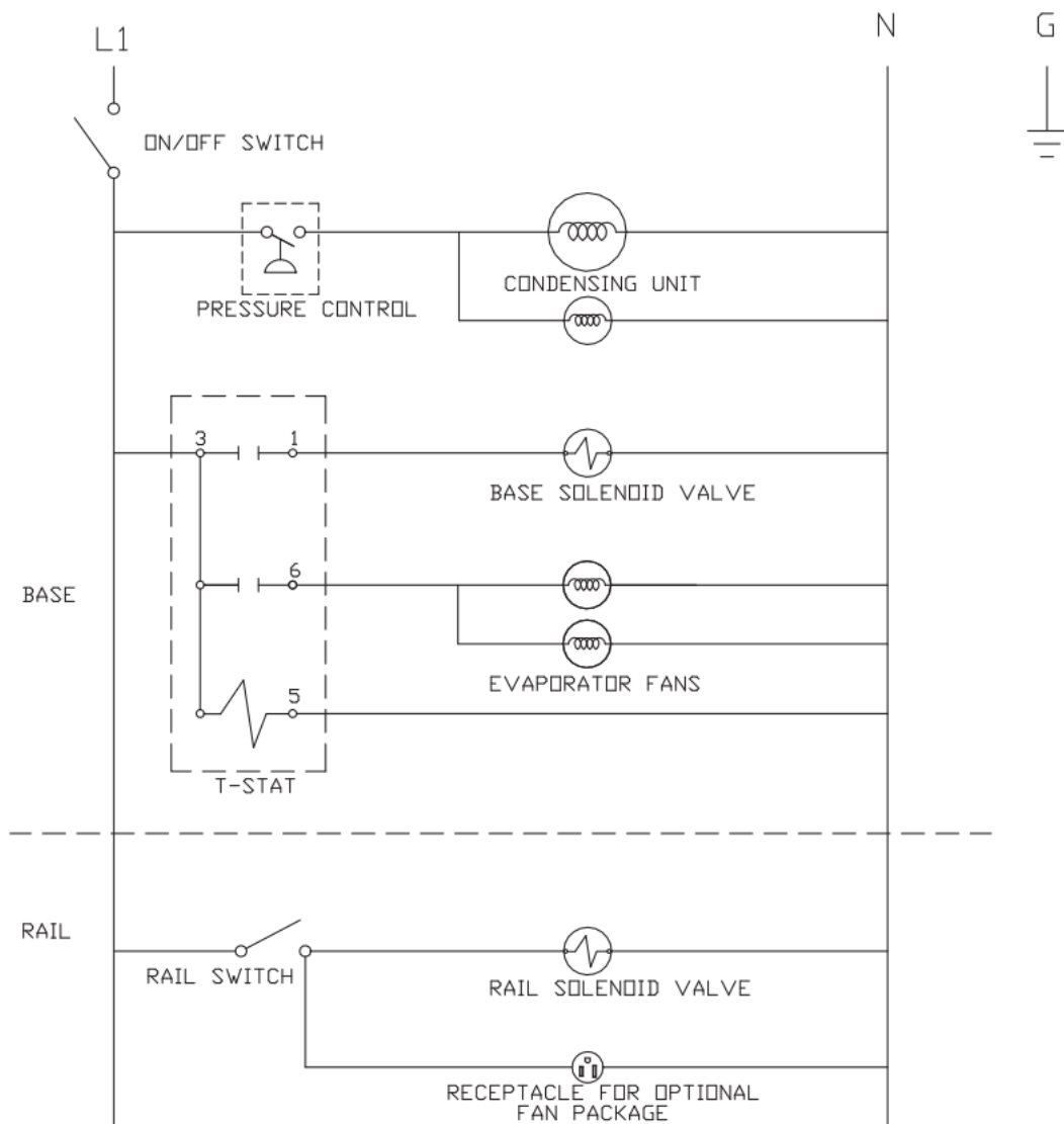
Wiring Diagram, F18MR, F18SR, F18DR & F18RR
