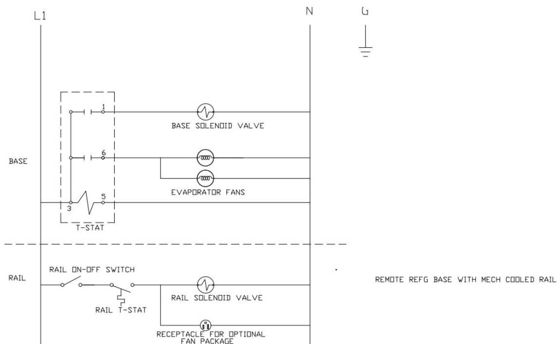
Wiring Diagram, F18FC
