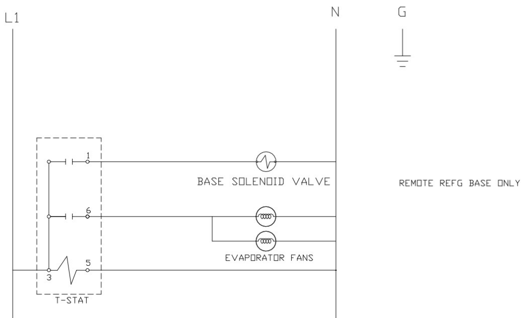
Wiring Diagram, F18MC, F18SC, F18DC & F18RC
