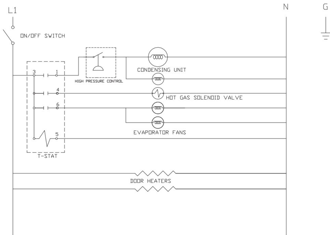
Wiring Diagram, F18FR
