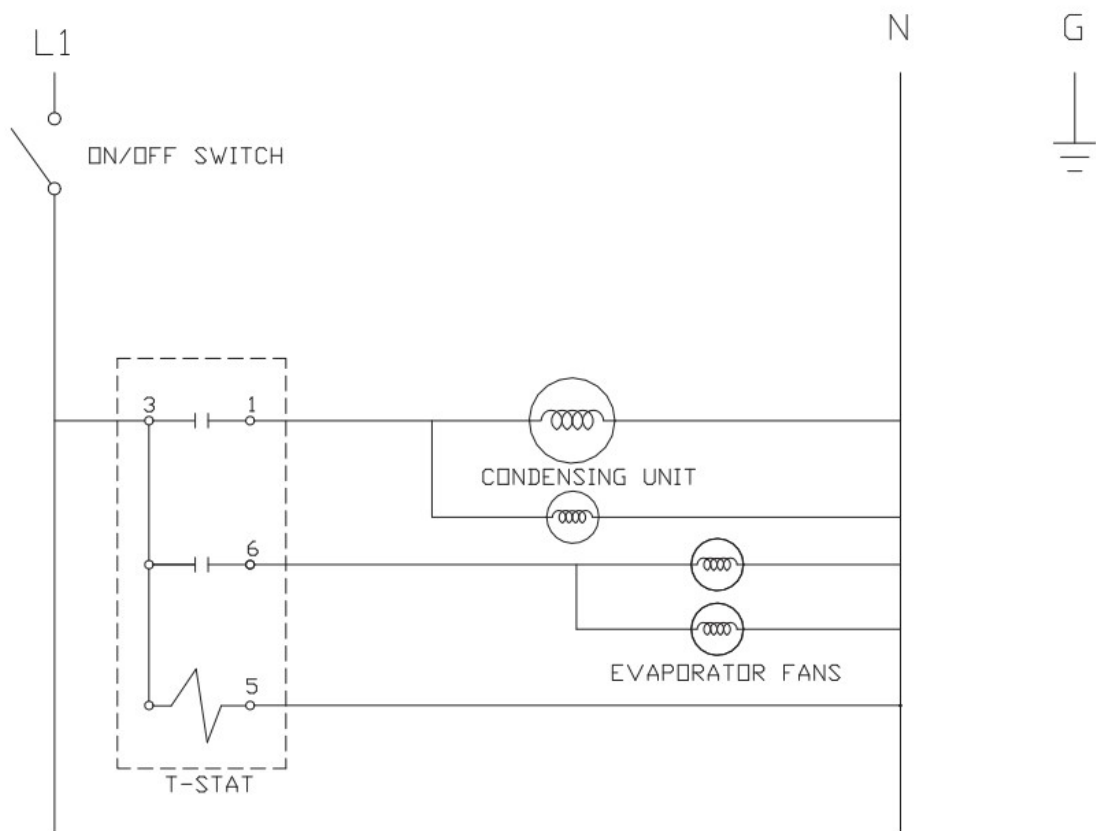
Wiring Diagram, F18WR
