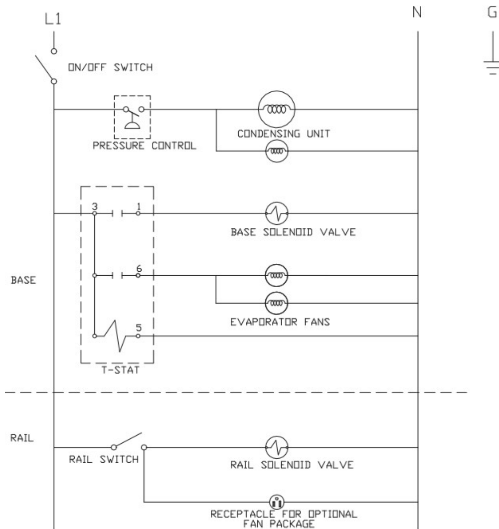
Wiring Diagram, F18MR, F18SR, F18DR & F18RR
