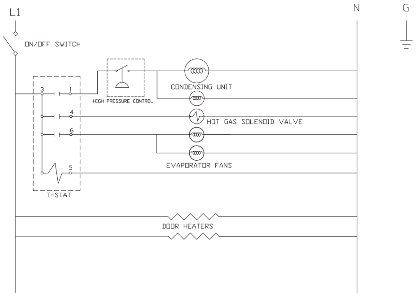
Wiring Diagram, F18FR
