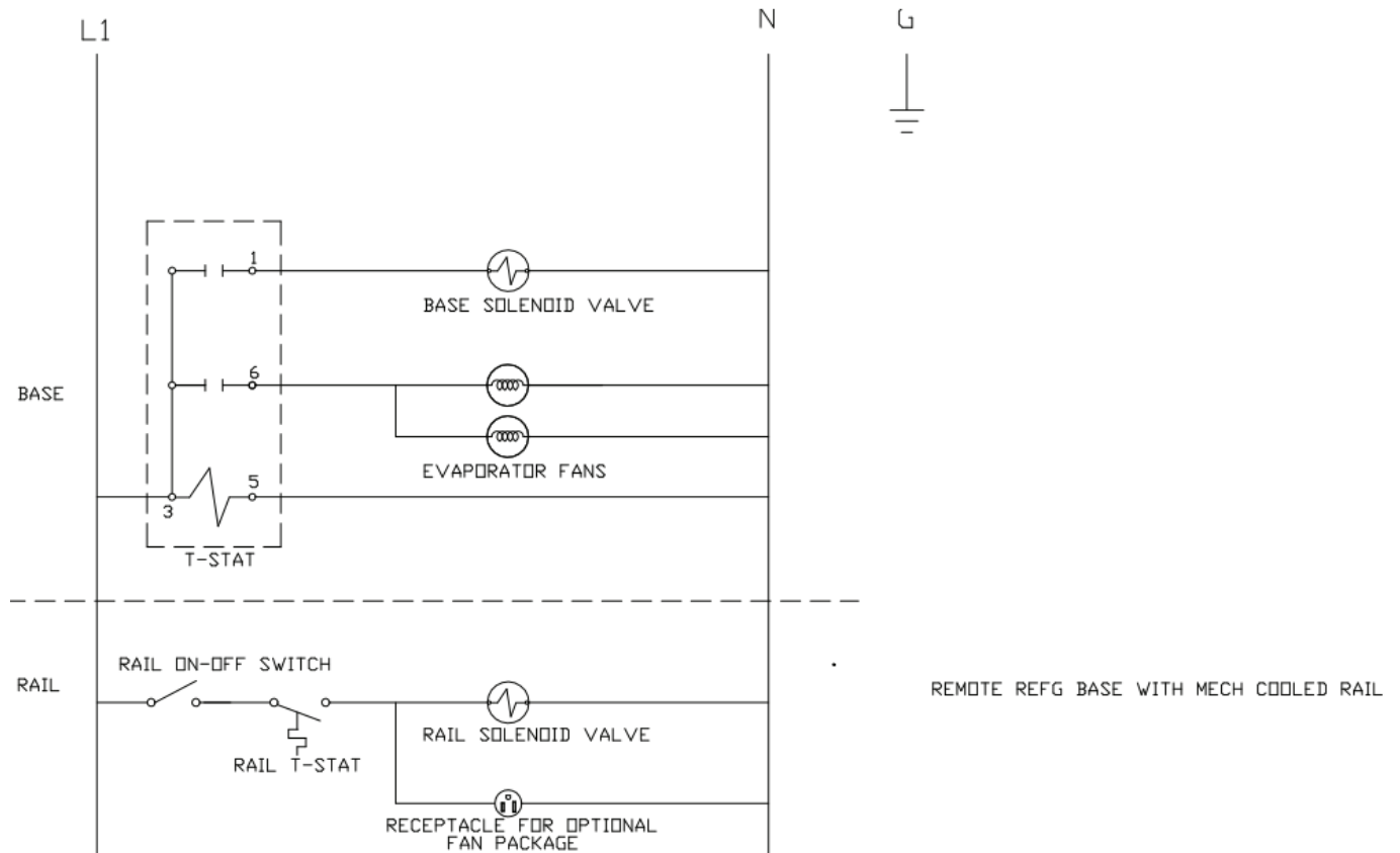
Wiring Diagram, F18FC
