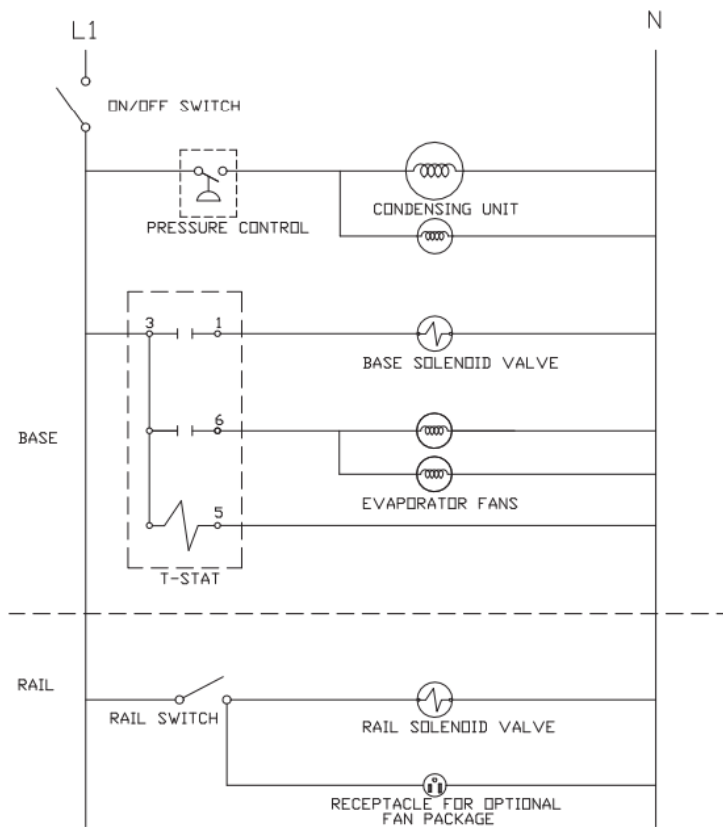
Wiring Diagram, F18MR, F18SR, F18DR & F18RR
