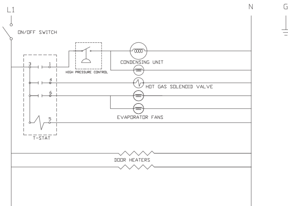
Wiring Diagram, F18FR
