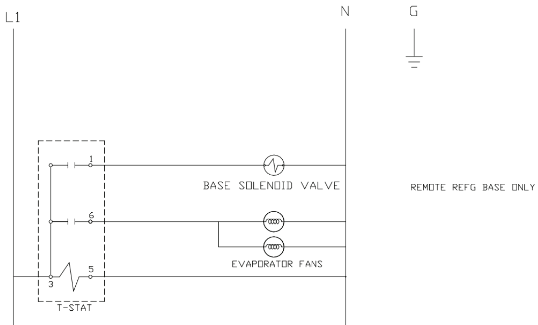
Wiring Diagram, F18MC, F18SC, F18DC & F18RC
