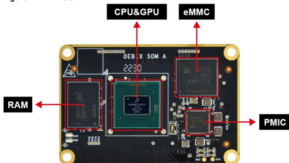
Figure 4 DEBIX SOM A
