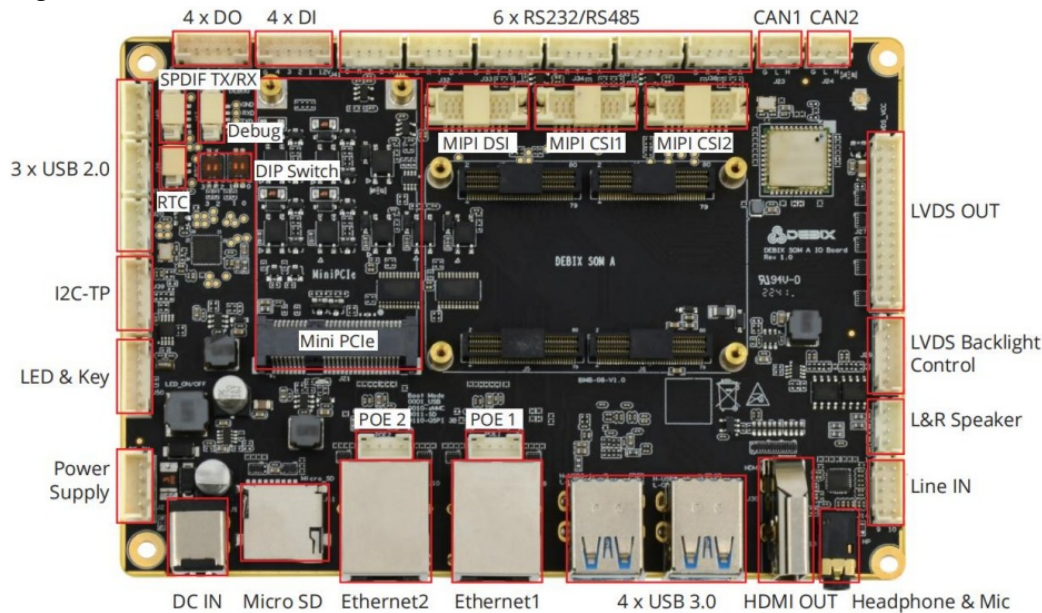
Figure 6 DEBIX SOM A I/O Board
