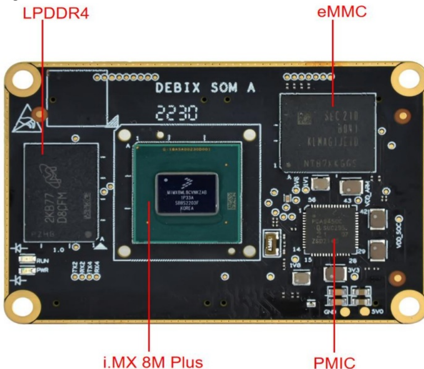
Figure 3 DEBIX SOM A Back
