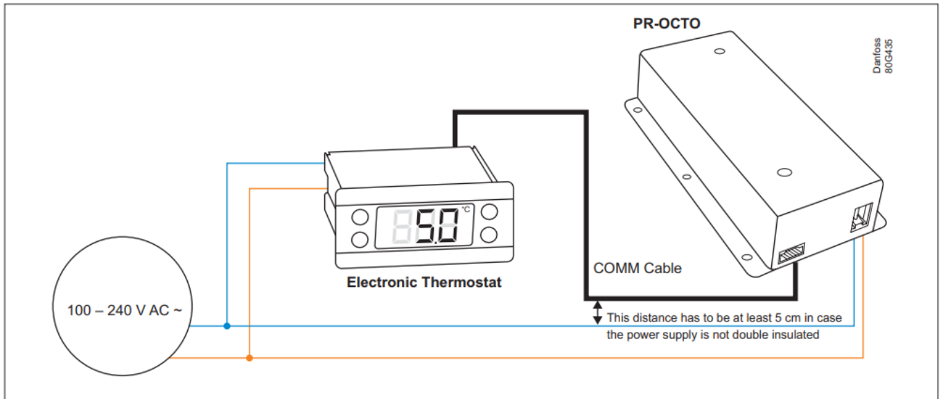
Fig. 3: Wiring details
