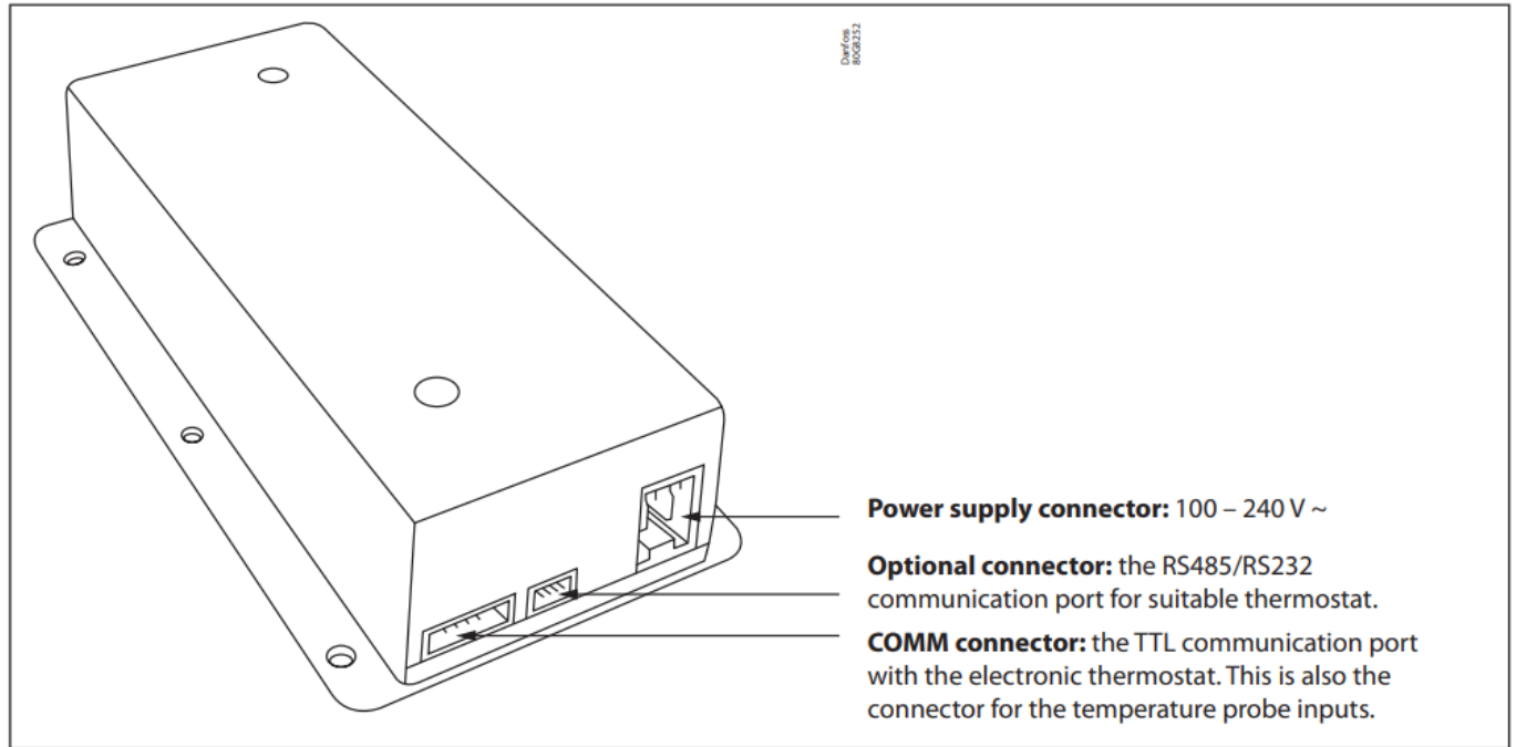
Fig. 2: Side B
