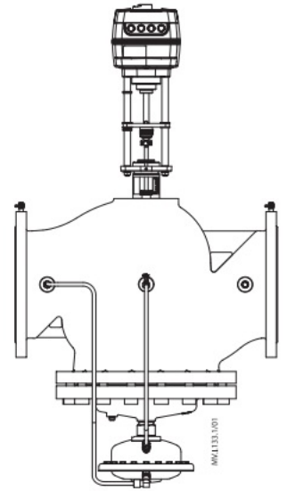
NovoCon® XL AB QM DN 200 - 250HF
