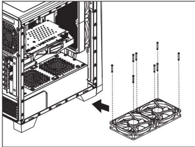
Install Fan
