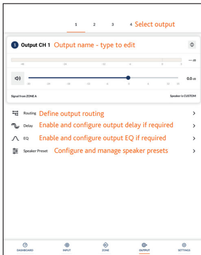
Diagram 5G Output Tab display
