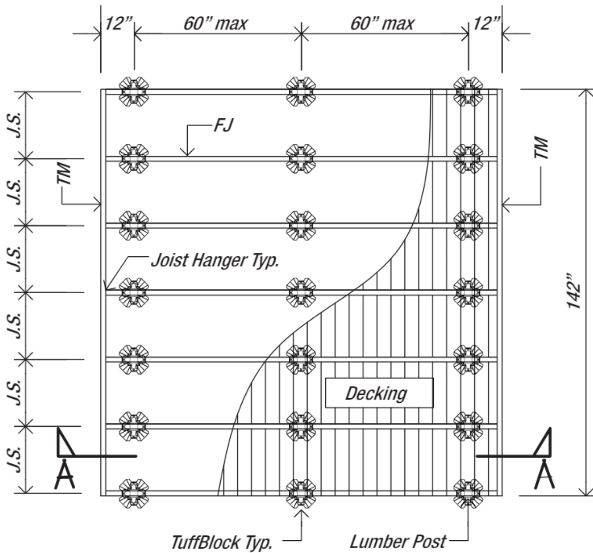
Section A-A
