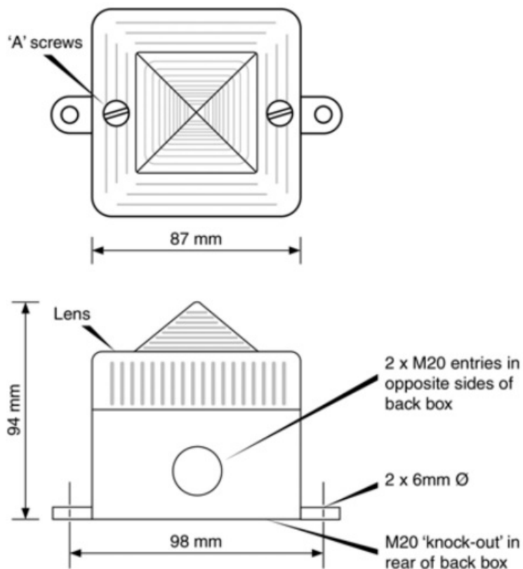
Fig 2 BA386 dimensions
