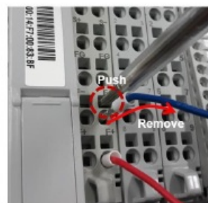
Remove cable
