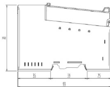
Module dimensions (mm)
