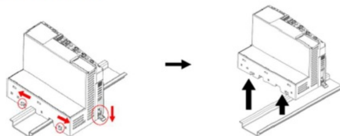
Dismount from DIN rail
