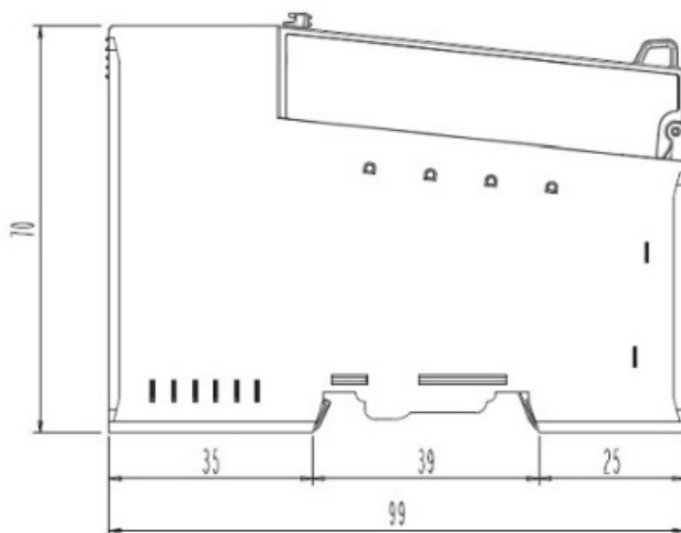
Module dimensions (mm)
