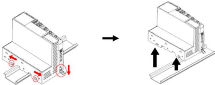
Dismount from DIN rail
