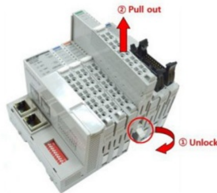
Dismount from DIN rail
