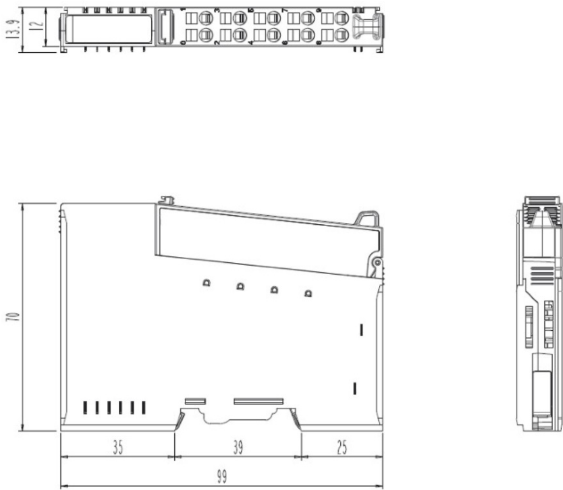
Module dimensions (mm)
