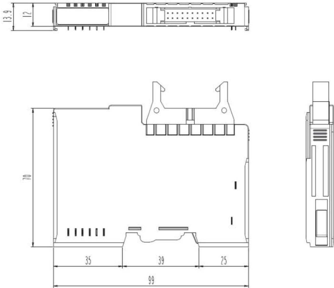
Module dimensions (mm)
