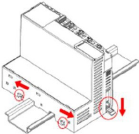
Dismount from DIN rail
