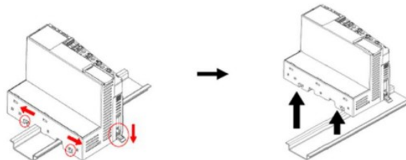
Dismount from DIN rail
