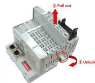
Dismount from DIN rail
