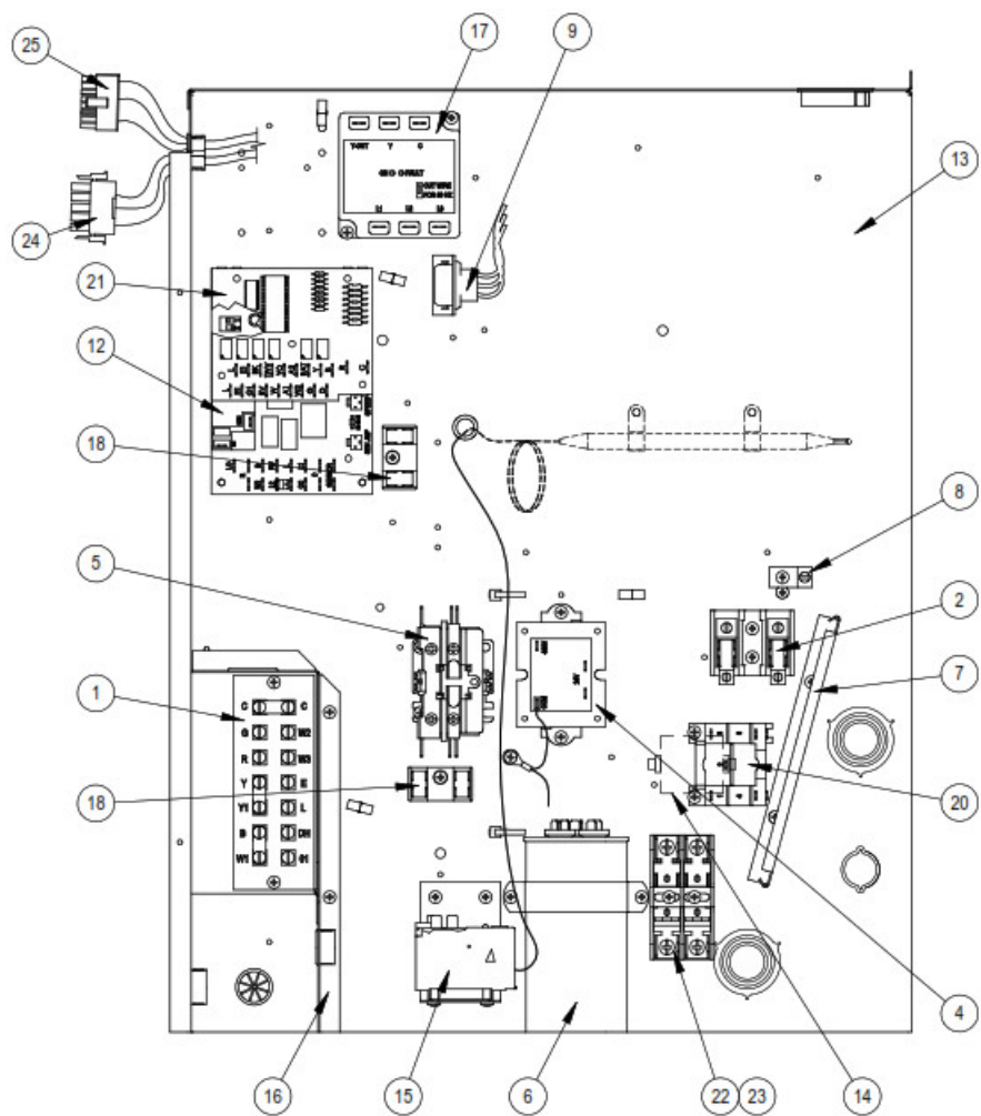
SXP-605
