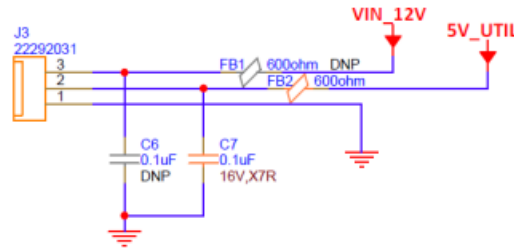
Figure 35 – Fan Header
