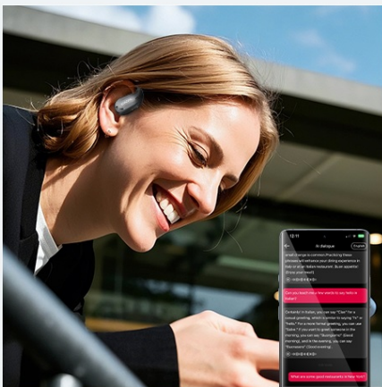
AI chat
