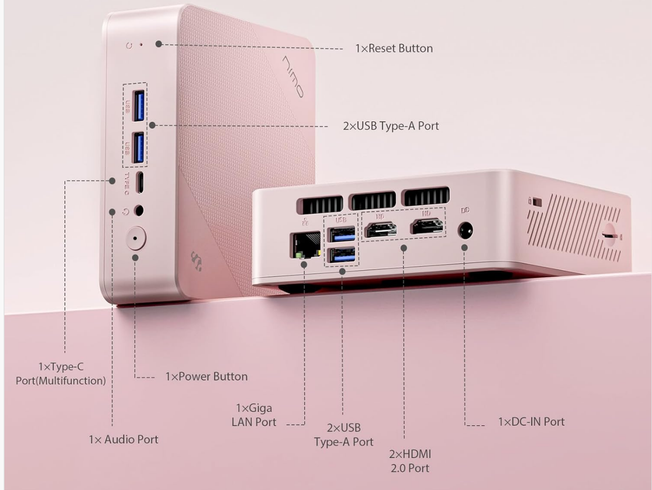
Figure 3.2: NIMO Mini PC N100 Port Layout
