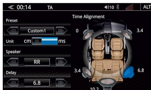
5-Kanal Laufzeitkorrektur
