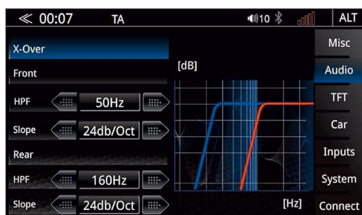
12 & 24 dB/Okt. Hoch- und Tiefpassfilter
