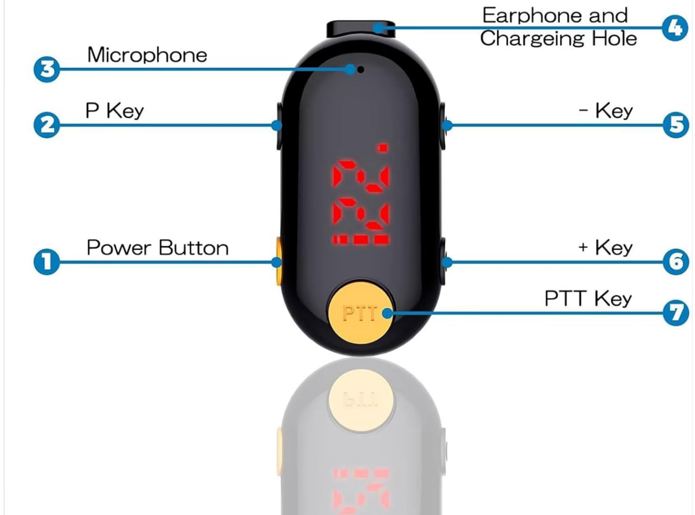
Image 2: Mini Walkie-Talkie Function Key Diagram.
