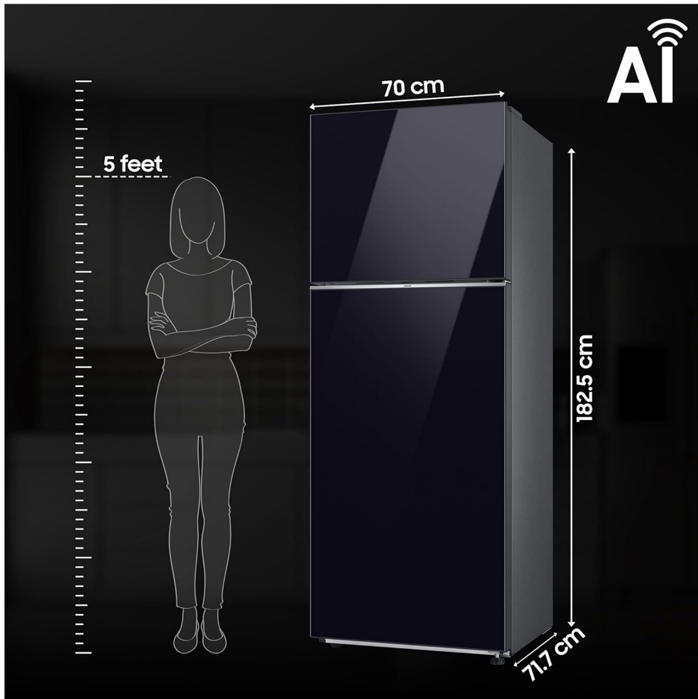
Image: Refrigerator dimensions: 71.7 cm (D) x 70 cm (W) x 182.5 cm (H).
