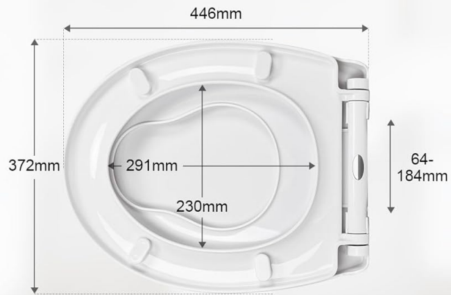
Dimensions du Siège de Toilettes
