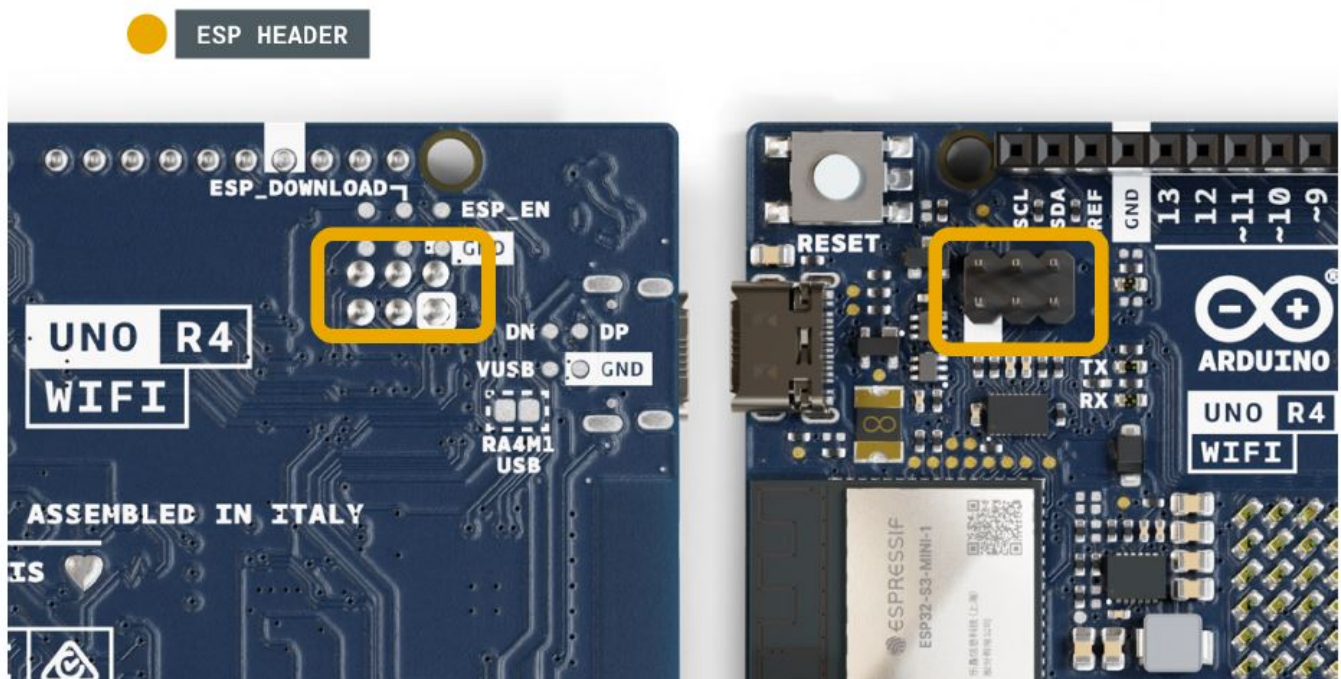
ESP header.
