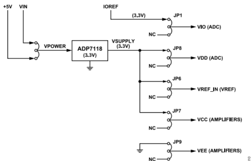
Figure 10. EVAL-AD4050-ARDZ/EVAL-AD4052-ARDZ Power Tree
