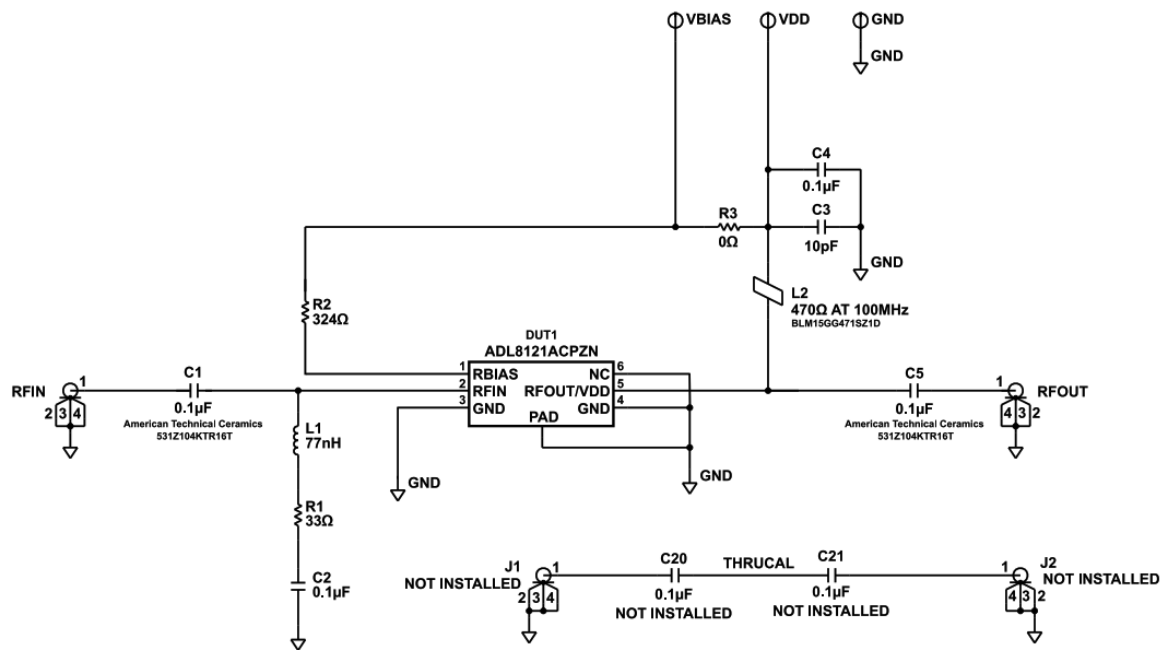
Figure 4. ADL8121-EVALZ Schematic
